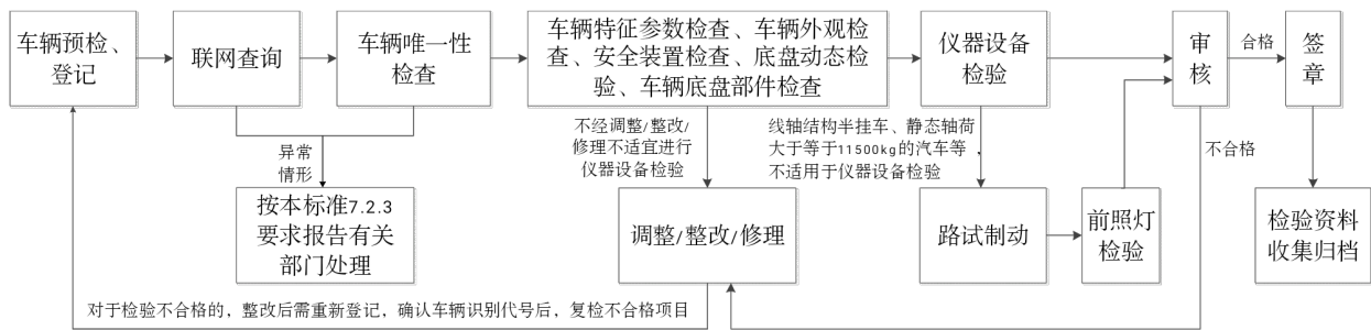
图A.1 机动车安全技术检验流程
